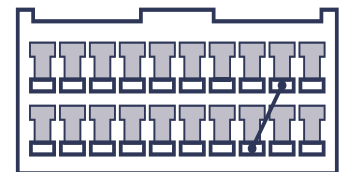
Рис. 15. Разъём иммобилайзера
